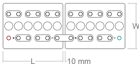
12V 1 OPzS 50-N6 to 12V 3 OPzS 150-N6
