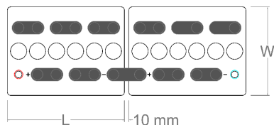
12V 1 OGiV 25-N7 to 12V 6 OGiV 150-N7
