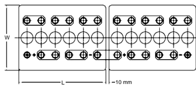
12V 1 OPzS 50-N6 to 12V 3 OPzS 150-N6
