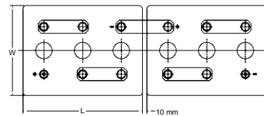
6V 3 OPzS 150-N6 to 6V 6 OPzS 300-N6
